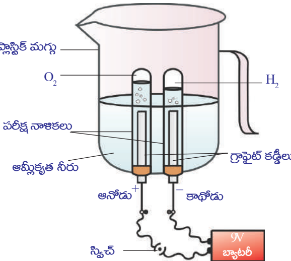
పటం-10: నీటి విద్యుద్విశ్లేషణం
