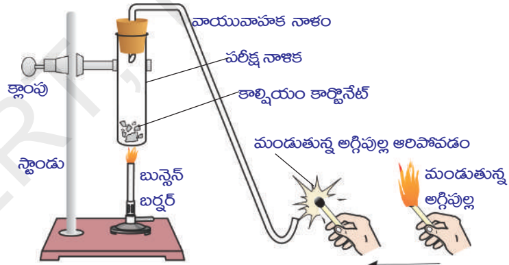
పటం-8: కాల్షియం కార్బోనేట్ ను వేడి చేసినప్పుడు
